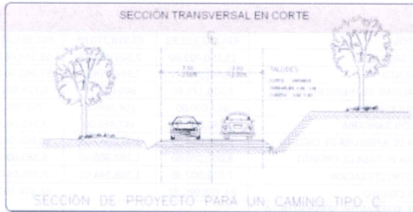
Figura 21. Sección transversal de los tramos
