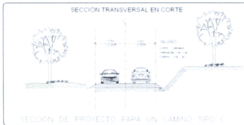
Figura 20. Sección transversal de los tramos
