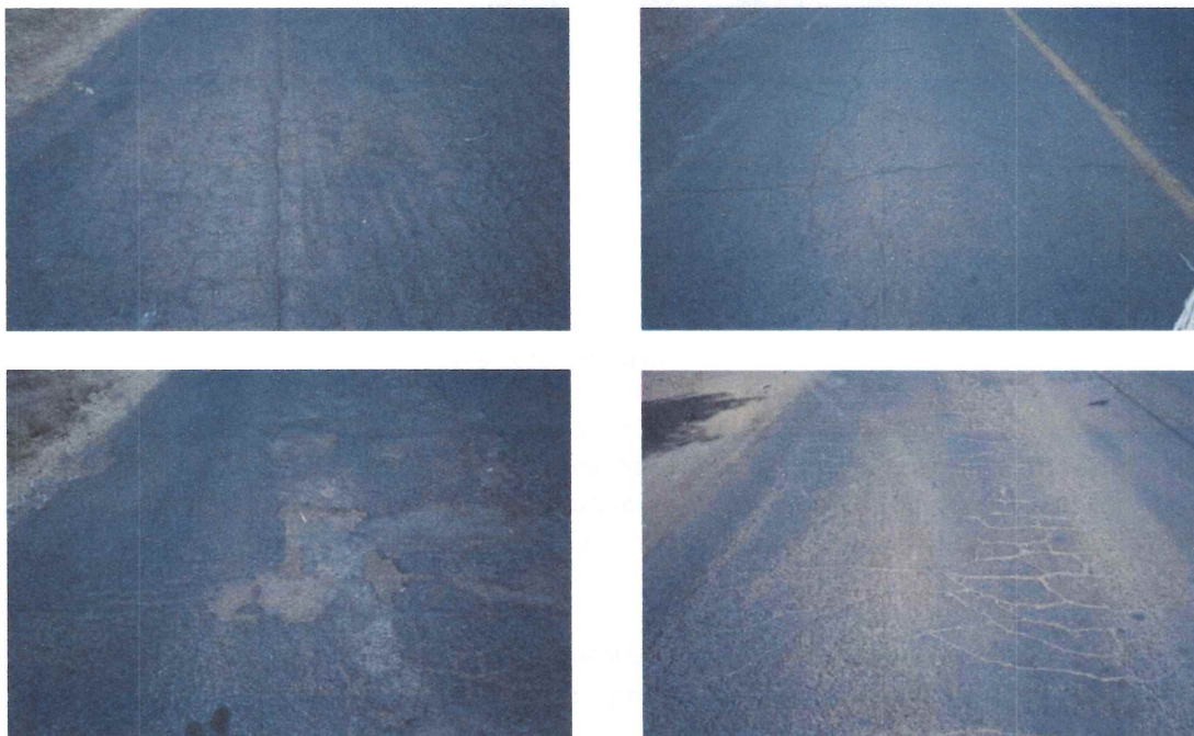
Figura 6. Deterioro en la superficie de rodamiento en las carreteras estatales MICH-04, MICH-07 y MICH-57 Toluca – Cotija – Puente Jaripo, Jacona – Peribán y Libramiento Sur de Zamora
