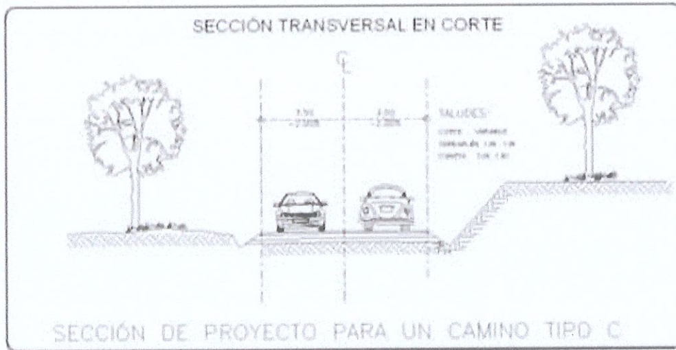
Figura 21. Sección transversal de los tramos
