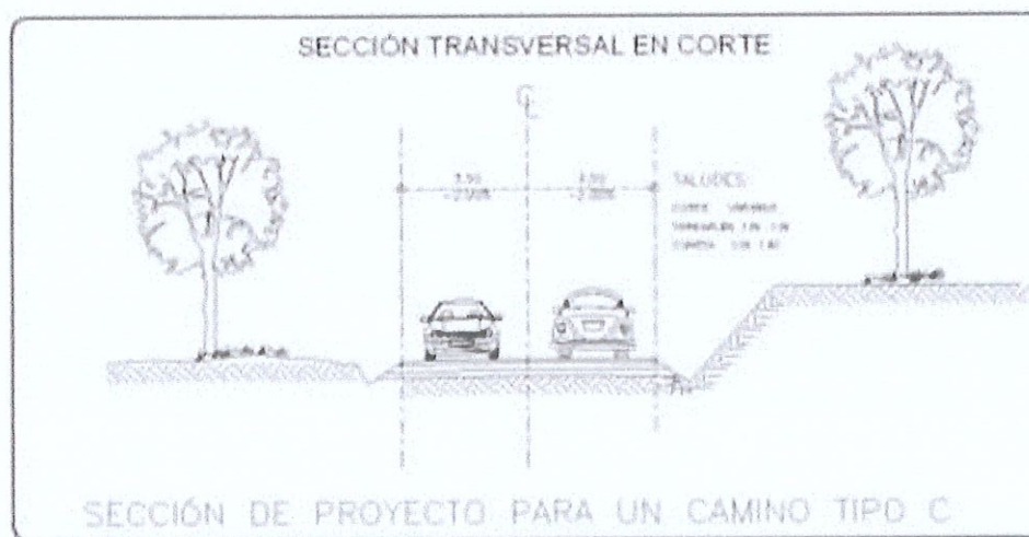
Figura 20. Sección transversal de los tramos
