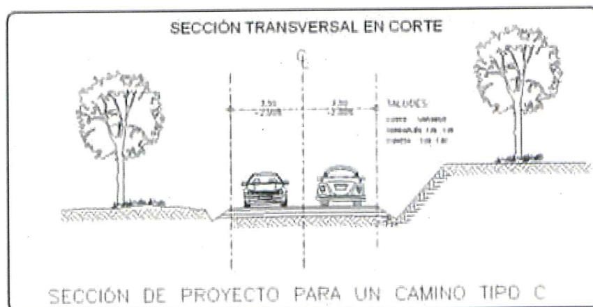
Figura 20. Sección transversal del tramo: Aguililla – Dos Aguas, del km 0+000 al km 13+680
