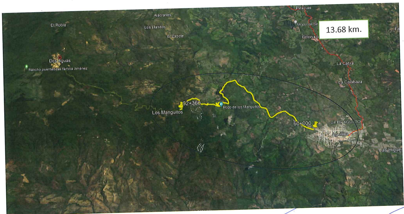
Figura 23. Ubicación regional de la Rehabilitación de la carretera Aguililla – Dos Aguas.
